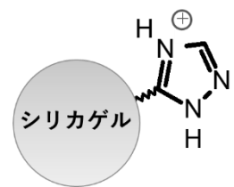
図 1 トリアゾール型固定相の模式図
