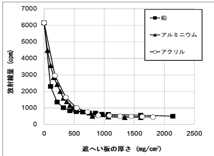
図2 鉛、アルミニウム、アクリルによる放射線の遮へい 縦軸はバックグラウンドを差し引いた放射線量 (cpm)、横軸は遮へい板の厚み (面密度 \text{mg}/\text{cm}^2 )。何もさえぎるものがないときに数千 cpm あった放射線が、遮へい板を線源の上に置いていくと減弱していく。減弱は、1000cpm あたりから緩やかになっている。
